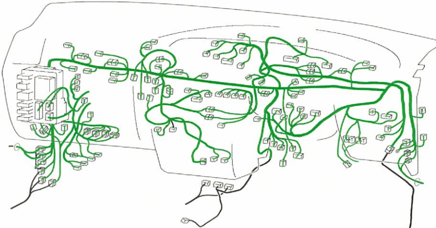
推奨除去部位:インパネワイヤハーネス
